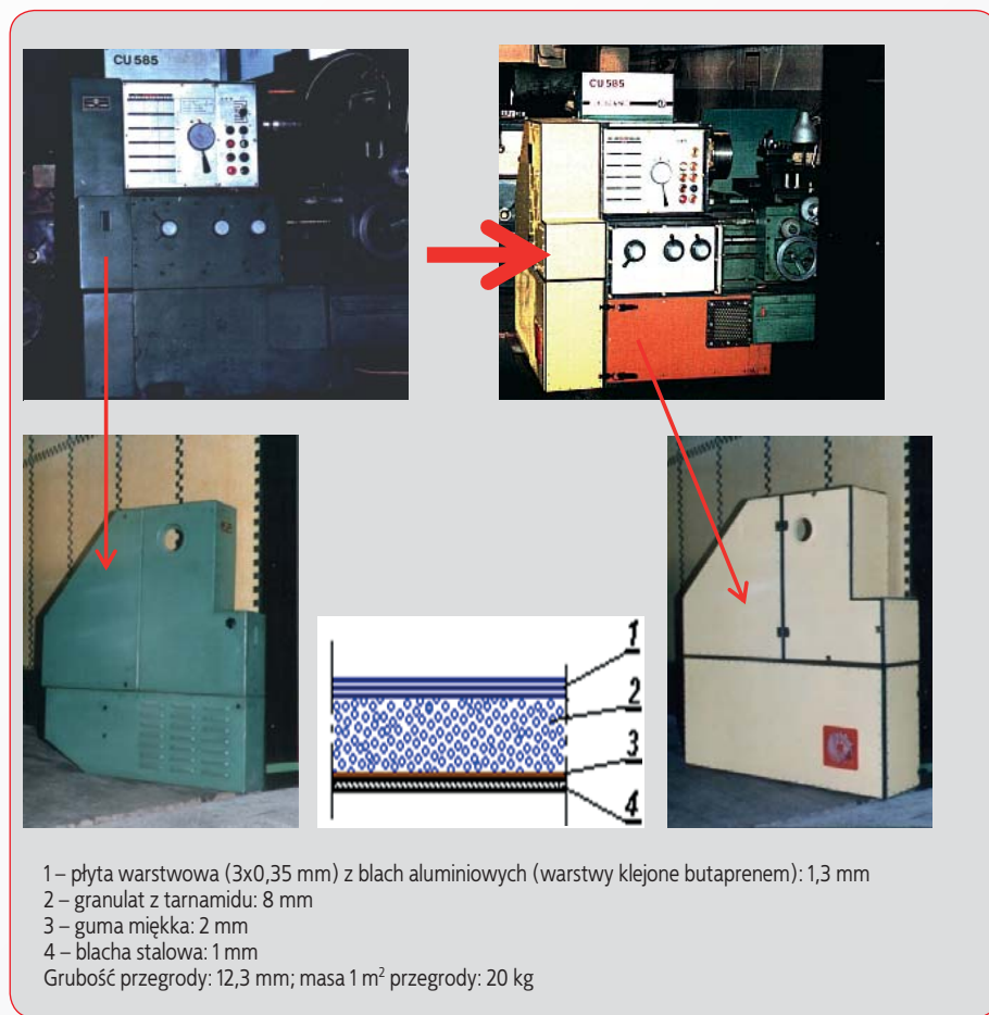
Rys. 12. Zmodyfikowana osłona boczna łańcuchów kinematycznych napędowych tokarki Fig. 12. Modified side cover of kinematic driving chains of a turning lathe
